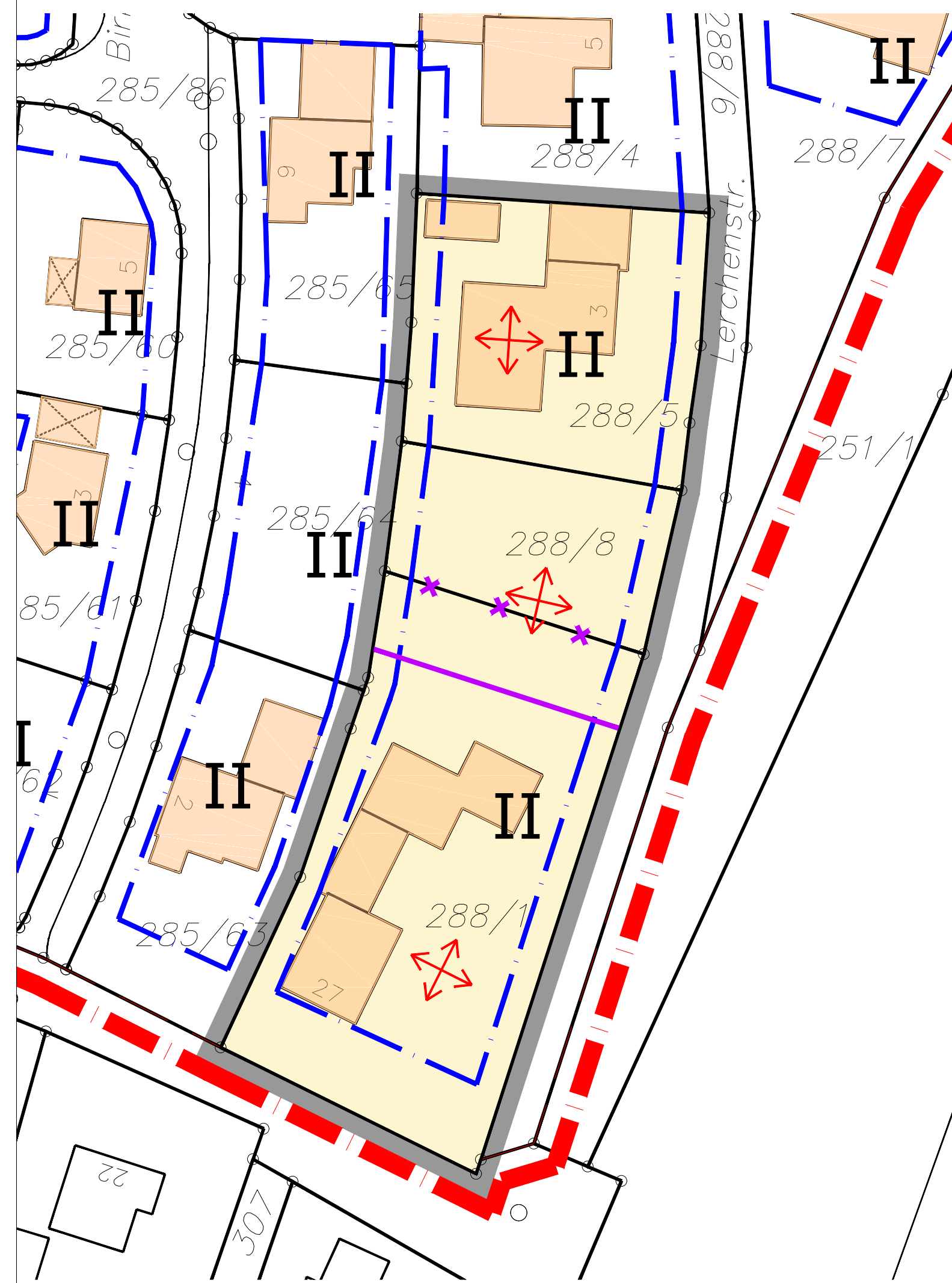
Planzeichnung, M 1:500
